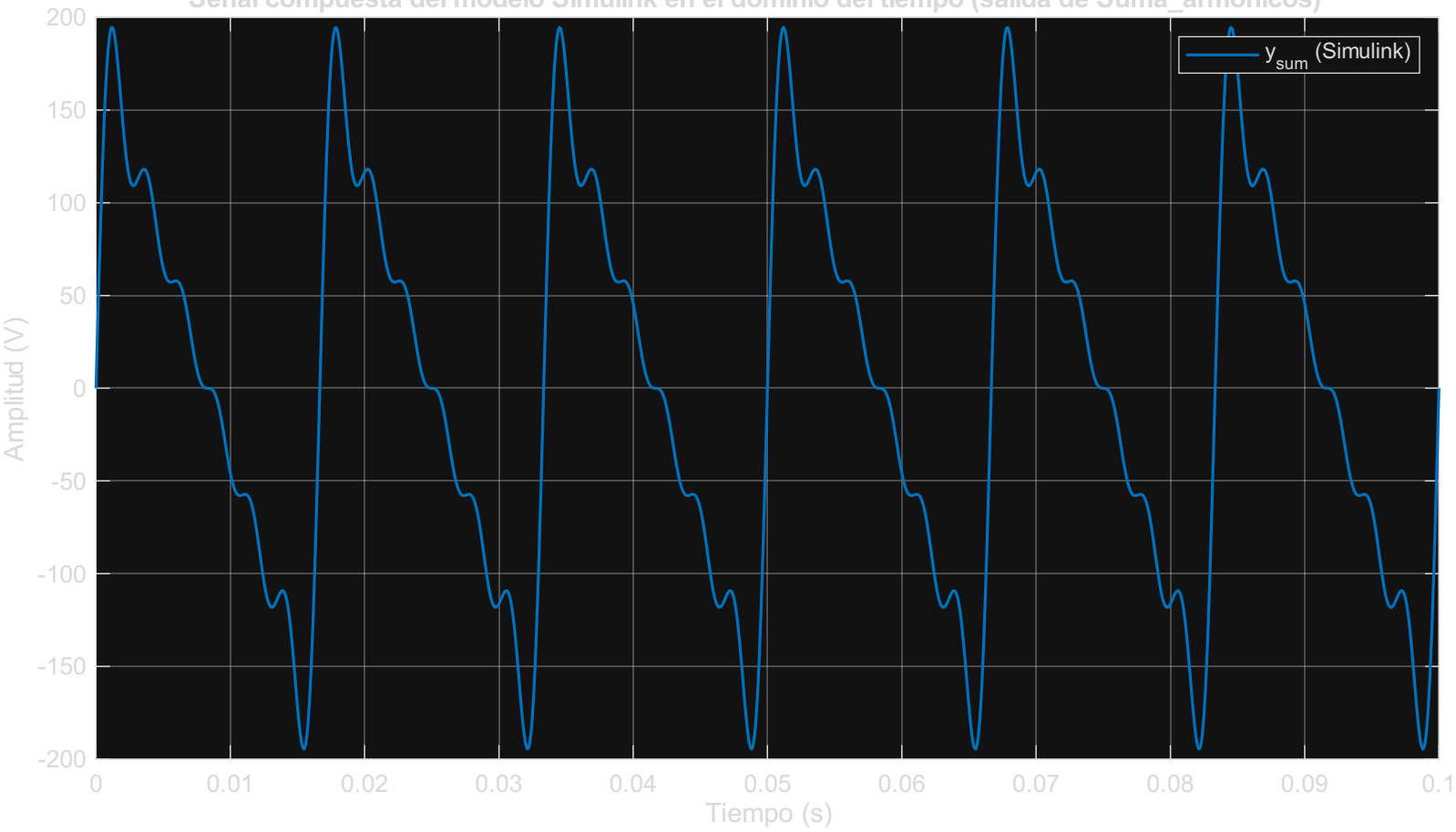
Señal compuesta del modelo Simulink en el dominio del tiempo (salida de Suma_armonicos)
